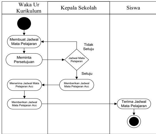
Gambar 1. Activity Diagram Informasi Jadwal Mata Pelajaran
