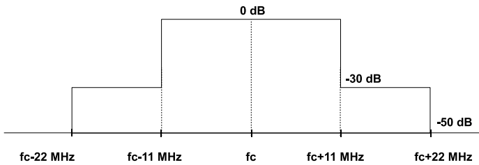
Fig. 2. IEEE 802.11 DSSS TSM.
