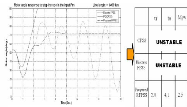
Fig. 8-d L=1400 km
