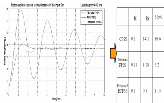
Fig. 8-b L=800 km
