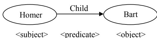
Fig. 2 RDF Triple
